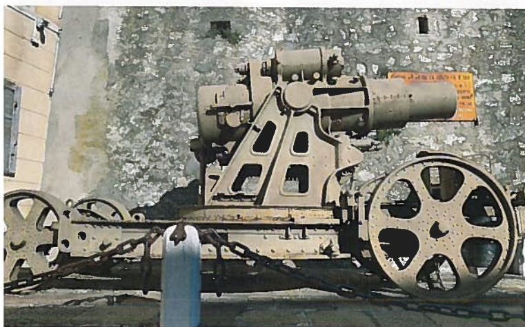
30,5-cm-M.11-Mörser, auch Škoda 305 mm Haubitze genannt.
